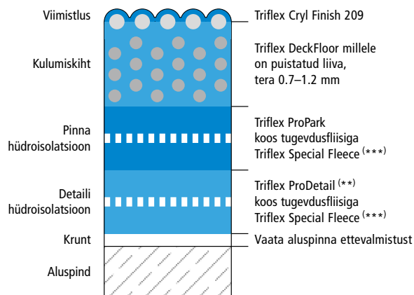
Süsteemi ülesehitus – Detail E
