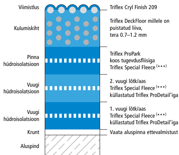
Süsteemi ülesehitus – Detail J
