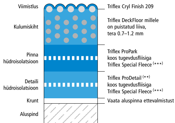
Süsteemi ülesehitus – Detail E
